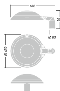
Thor S - montage en top
