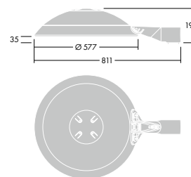
Thor L - montage latéral
