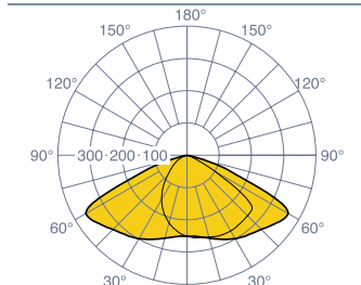
Thor L - montage latéral
