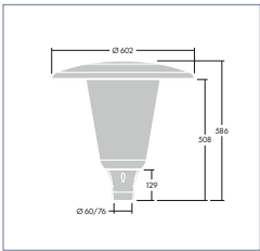
BREITE VERSION Ø 60 UND Ø 76
