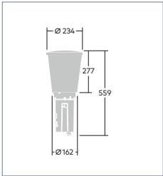
MASTAUFSATZLEUCHTE CANDLE
