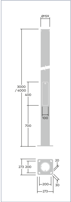
SÄULE CANDLE
